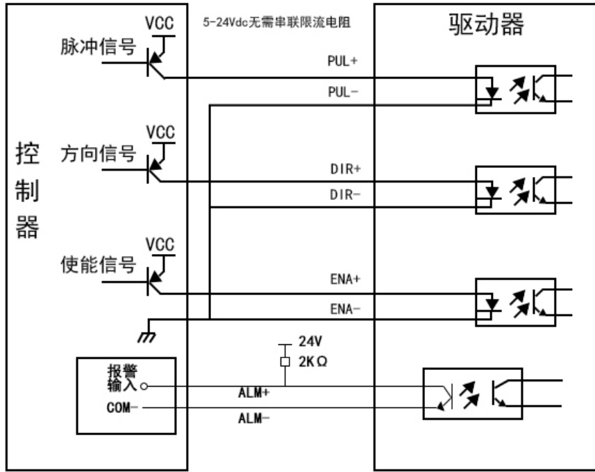
共阴极接法
