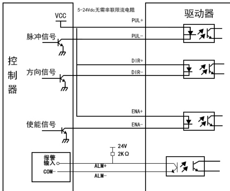
共阳极接法
